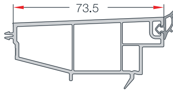
EŞİK KAPAMA PROFİLİ THRESHOLD CLOSING PROFILE AKS 1145
