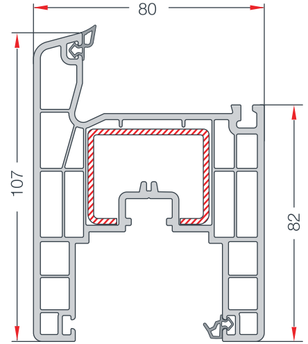
MASTERLINE SÜRME KANAT PROFİLİ MASTERLINE SLIDING SASH PROFILE EN 343
