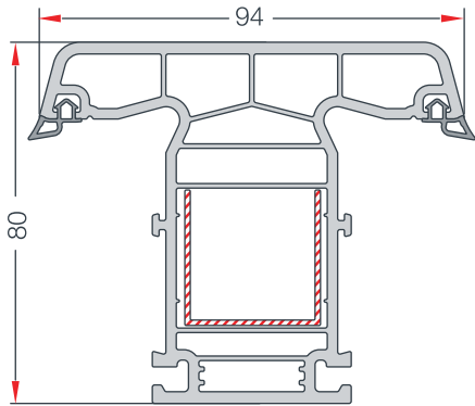
ORTA KAYIT PROFİLİ MULLION PROFILE EN 72
